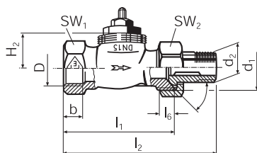
Термостатический клапан торцевого соединения (Торцевой клапан) 2310/2311; 2340/2341; 3513/3514
