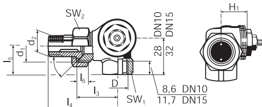
Термостатический клапан торцевого соединения (Торцевой клапан) 2312/2313; 2342/2343; 3533/3534
