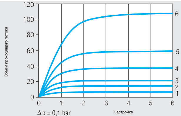
Оптимальное разграничение площади проходного сечения потока в системе отопления
