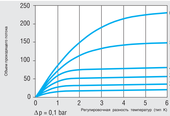
Оптимальное разграничение площади проходного сечения потока в системе отопления
