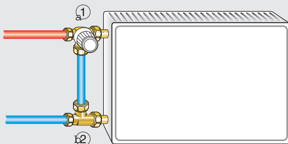
1. Термостатический трехходовой клапан с автоматическим регулированием байпаса 2. Байпас T-образной формы
