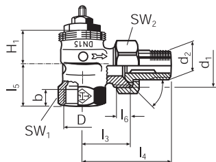
Термостатический клапан осевого соединения (Осевой клапан) 2225; 2245; 3430; 3511.
