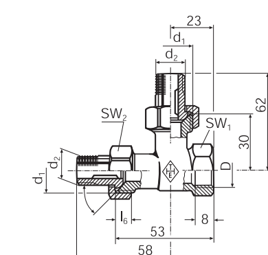
Термостатический клапан тройник (байпасный) (байпасный клапан) 4144; 4145; 4154; 4155; 4156
