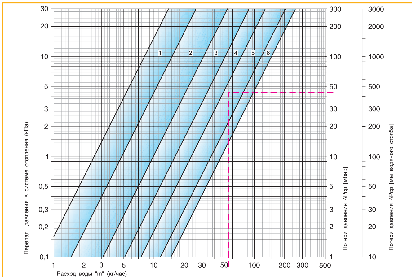
Диаграмма, клапан с термостатической головкой
