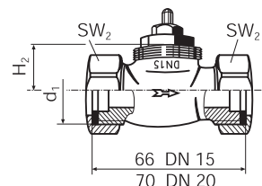
Термостатический клапан прямого соединения с прокладками плоского сечения (Прямодный клапан) 2072; 2074; 2076.
