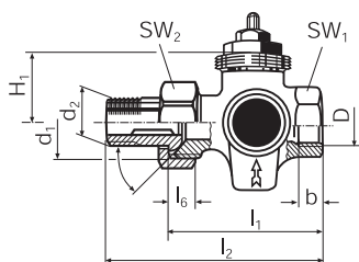
Термостатический клапан трехходового (байпасного) соединения (байпасный клапан) 4138; 4139; 4140/4141; 4142/4143
