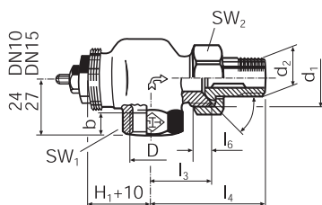
Термостатический клапан осевого соединения (Осевой клапан) 2235; 3530
