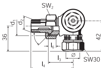
Термостатический клапан тройник (байпасный) (байпасный клапан) 4144; 4145; 4154; 4155; 4156
