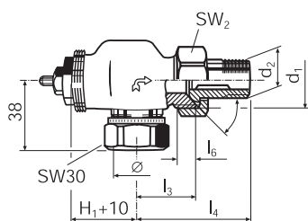
Термостатический клапан осевого соединения (Осевой клапан) 2235; 3530
